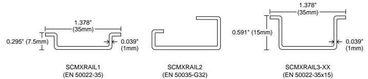
FIGURE 25. DIN Rail Styles.
